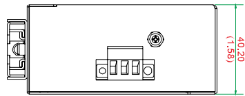
顶视图
