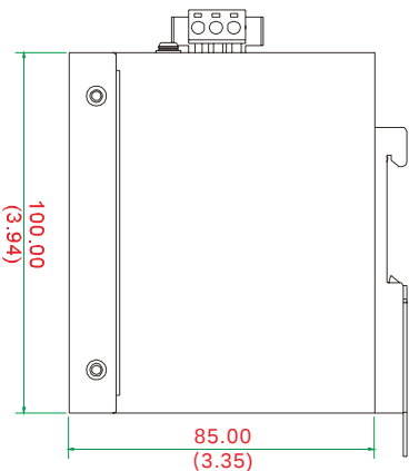
左侧视图
