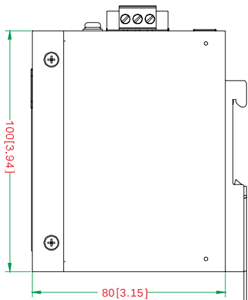
左侧视图
